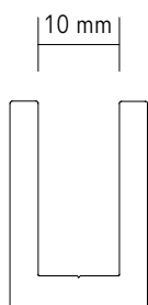
Extrusions pour écran en feutre 3/8" / 3/8" felt screen extrusions
