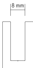
Extrusions pour écran en verre 1/4" / 1/4" glass screen extrusions
